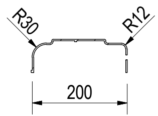
A-A (1:8)
